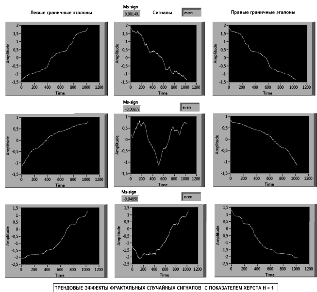
Рис. 3. Пример сравнения трендов фрактальных сигналов
