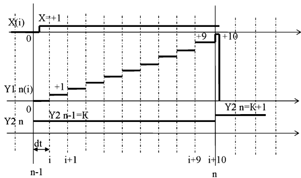
Рис. 3. Временная диаграмма работы двойного интегратора при единичном воздействии на входе интегратора
