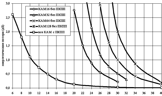
Рис. 6. Зависимость энергетических потерь от отношения сигнал/помеха
