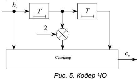
Рис. 5. Кодер ЧО
