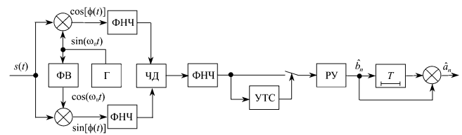
Рис. 8. Некогерентный демодулятор сигналов CQPSK на основе частотного детектора
