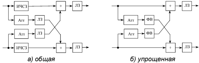
Рис. 4. Структурные схемы двухканальной модели радиоканала
